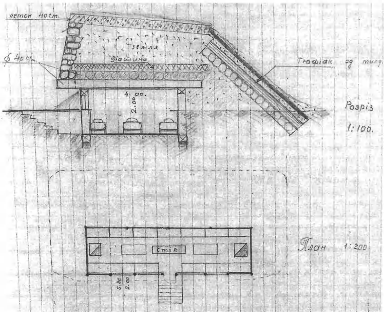
Землянка з покриттям і забезпеченням з тилу і боків од гранат 10 см і бомб льотничих до 150 кг
